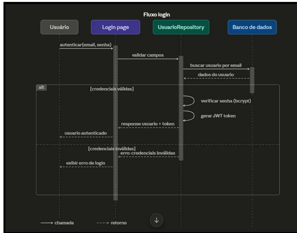
Figura 38 – Diagrama de sequência - Fluxo login da Safety Intelligence.
