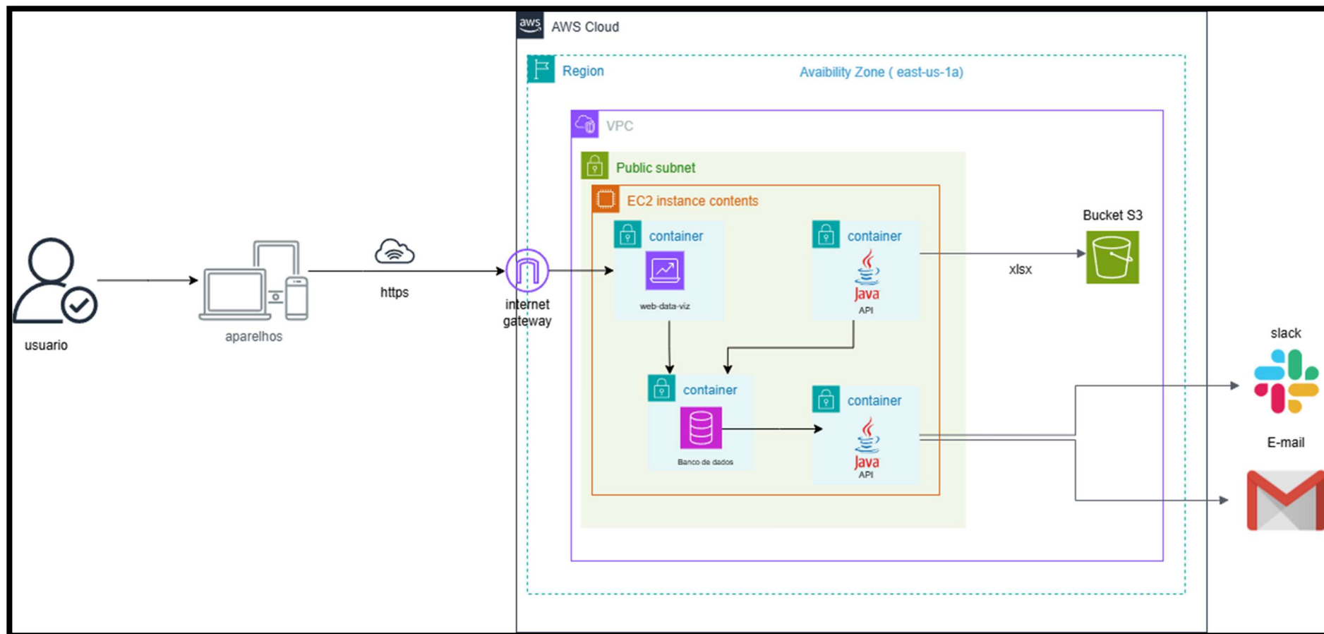
Figura 31 – Arquitetura da Solução da Safety Intelligence.
