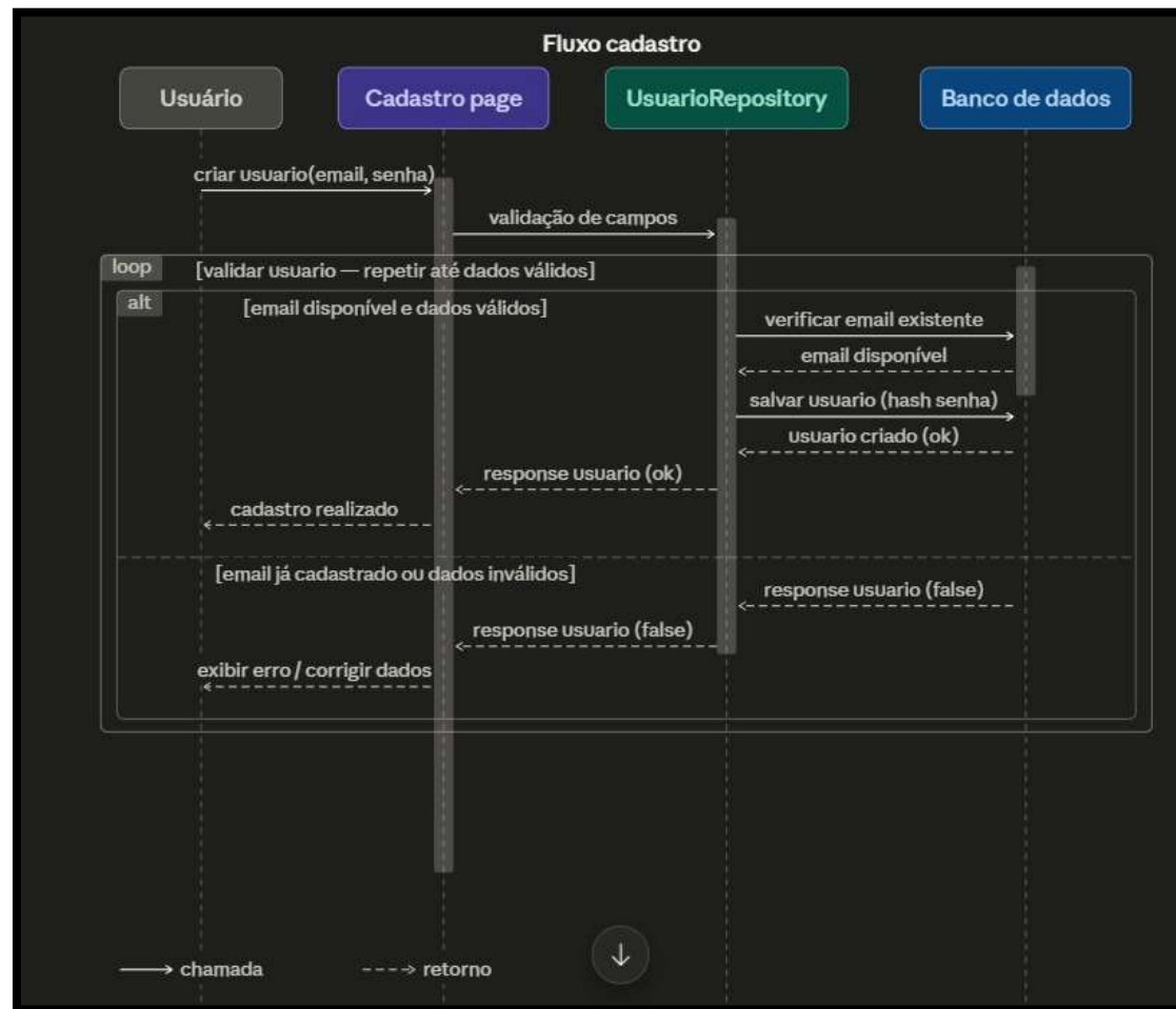
Figura 37 – Diagrama de sequência - Fluxo cadastro da Safety Intelligence.
