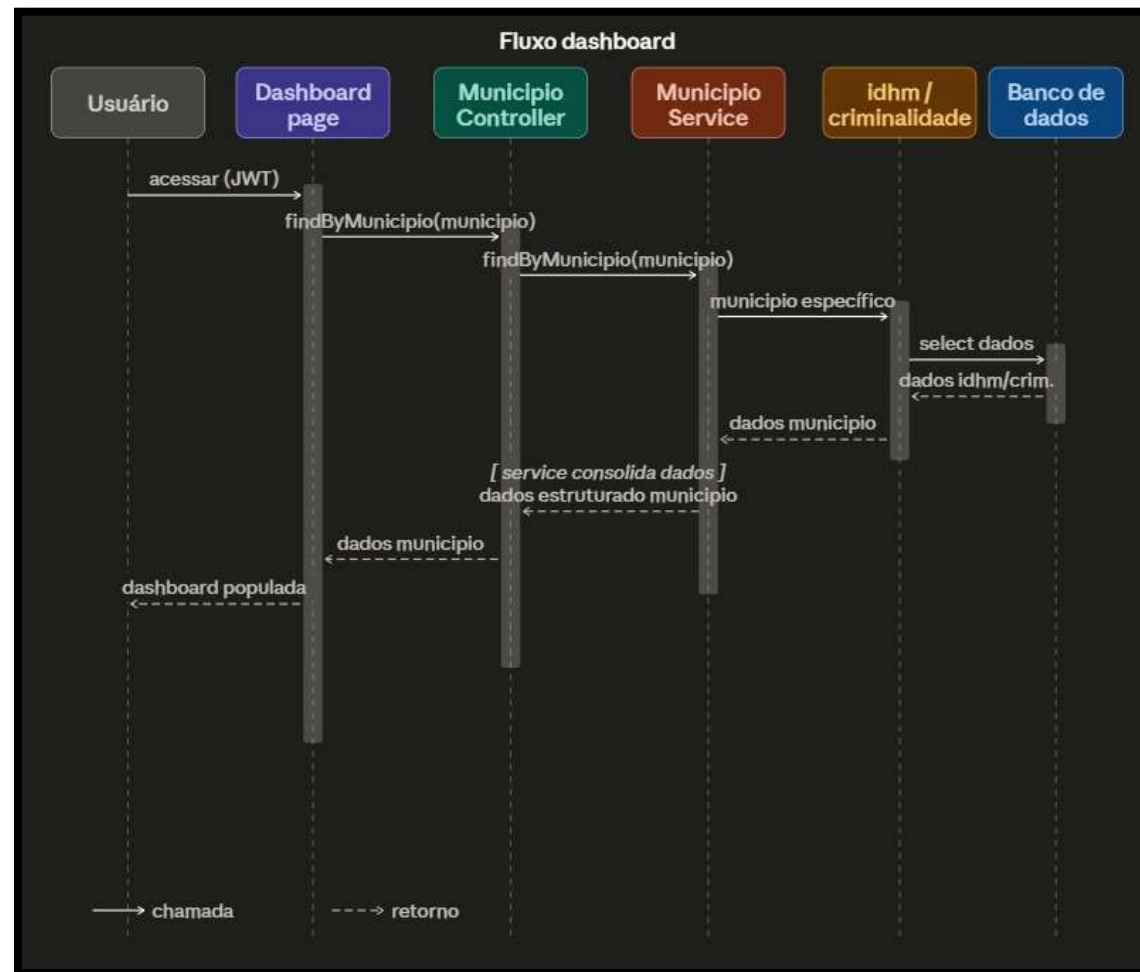
Figura 39 – Diagrama de sequência - Fluxo dashboard da Safety Intelligence.
